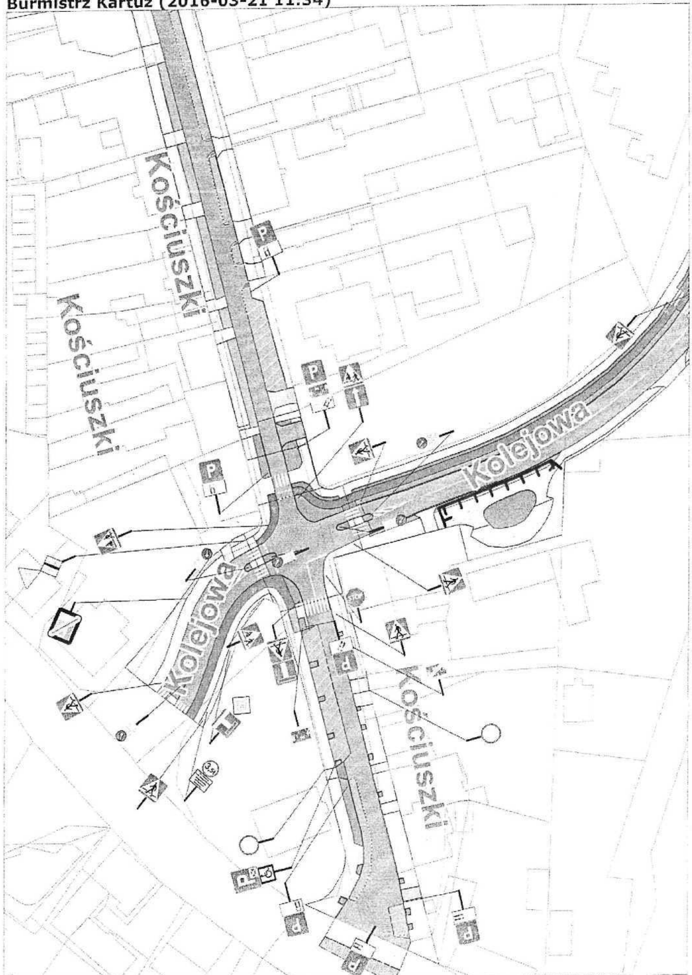
Wydruk wygenerowany za pomocą programu RoadMan. (1:1000)
