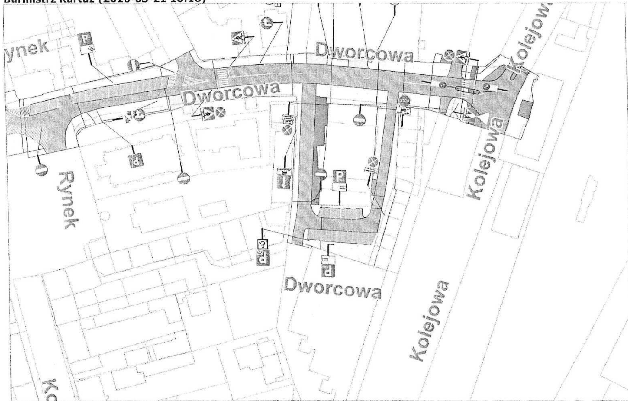
Wydruk wygenerowany za pomocą programu RoadMan. (1:1000)
